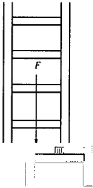
图 B.7 垂直挠度试验布置图
