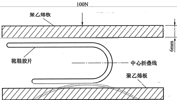
图 2 耐低温试验
